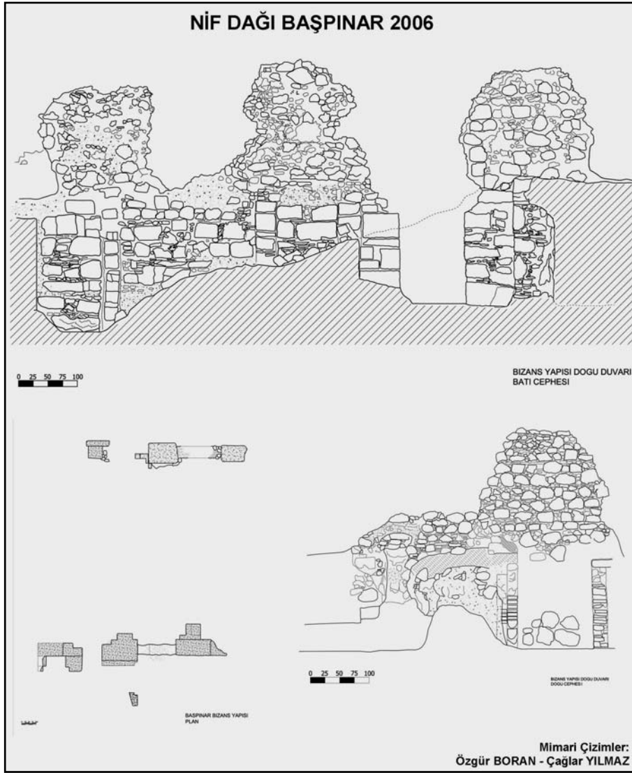
Resim 14: Nif Dağı - Başpinar 2006 Bizans yapısı plan ve rölövesi
